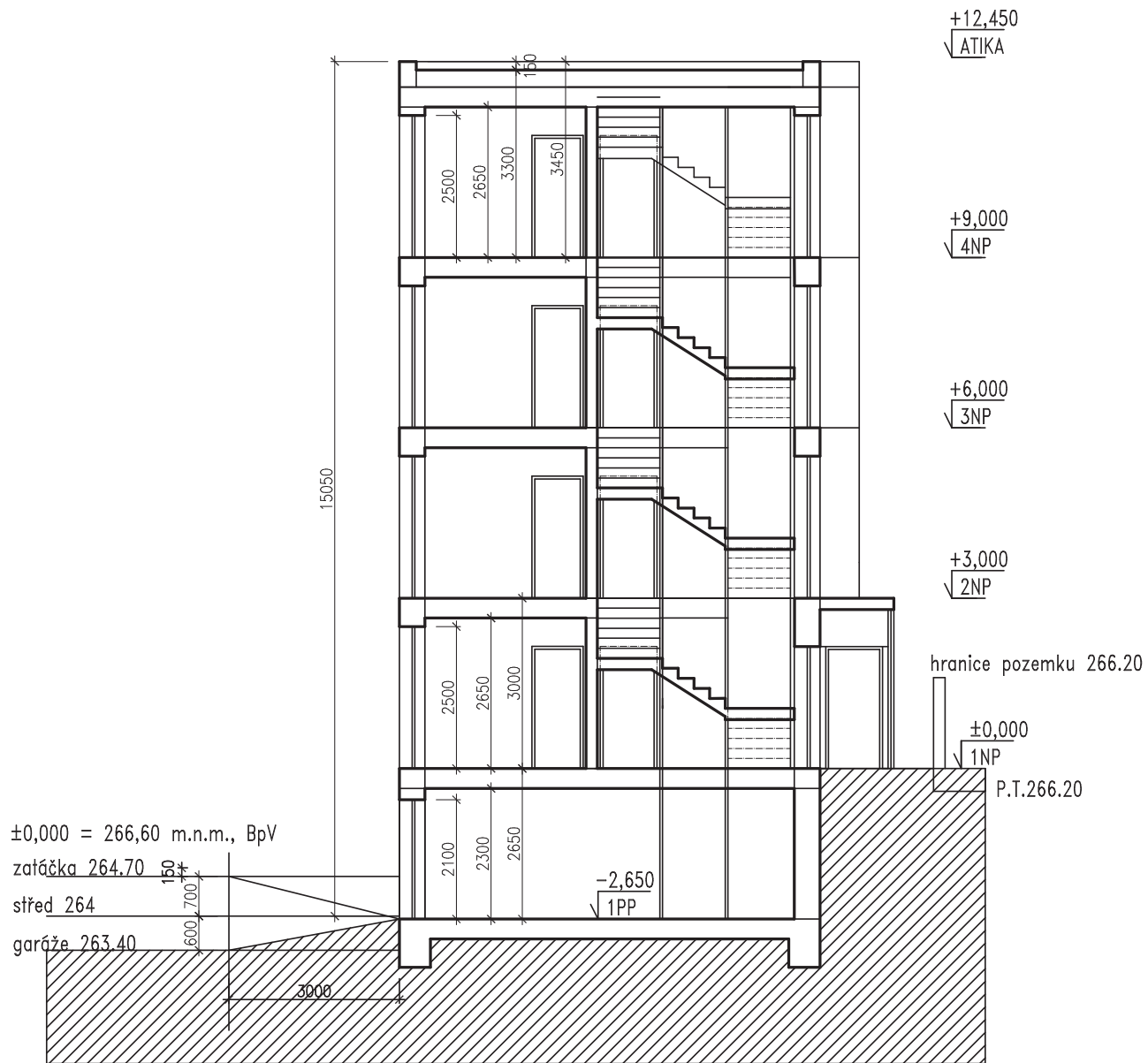
PŘÍČNÝ ŘEZ
